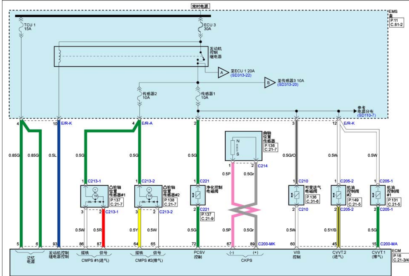
发动机控制系统(G4NA : NU 2.0L MPI M/T)(3)
